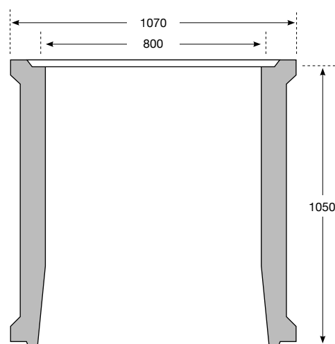
ÉLÉMENT DE 1050
