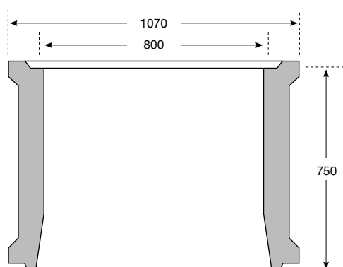
ÉLÉMENT DE 750
