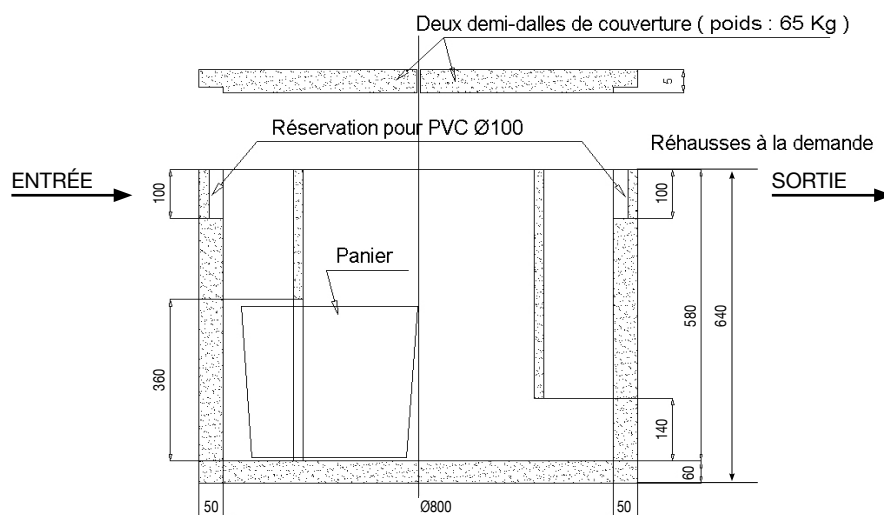
COUPE AA
